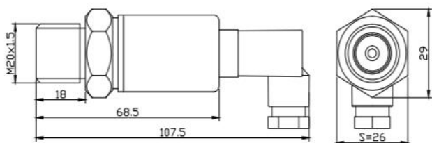
尺寸图：
